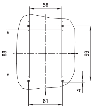
Монтажные размеры
