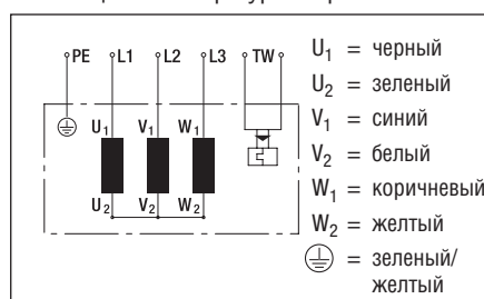
5b) Схема «звезда» (низкое значение частоты вращения) с выведенными концами температурного реле
