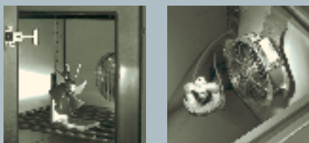
Слева: камера для климатических испытаний Справа: установка для испытаний в солевом тумане
